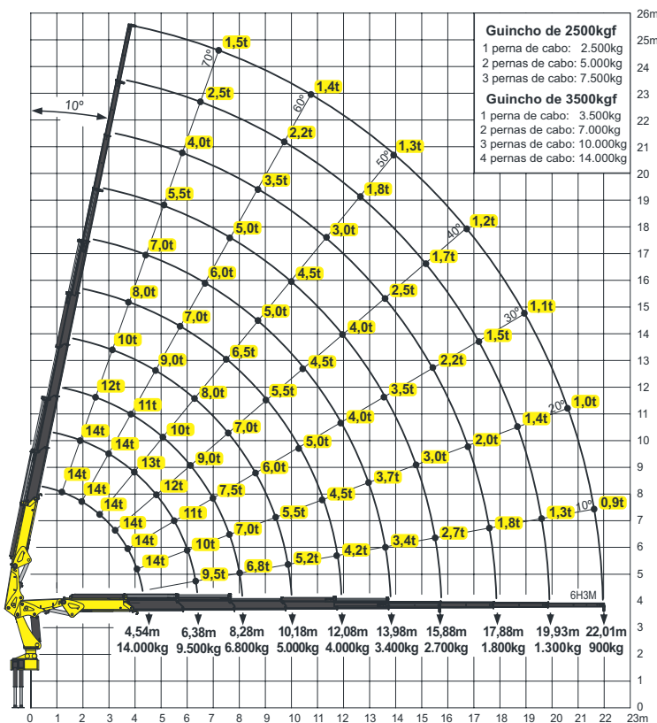
Gráfico de carga com Fly-Jib
