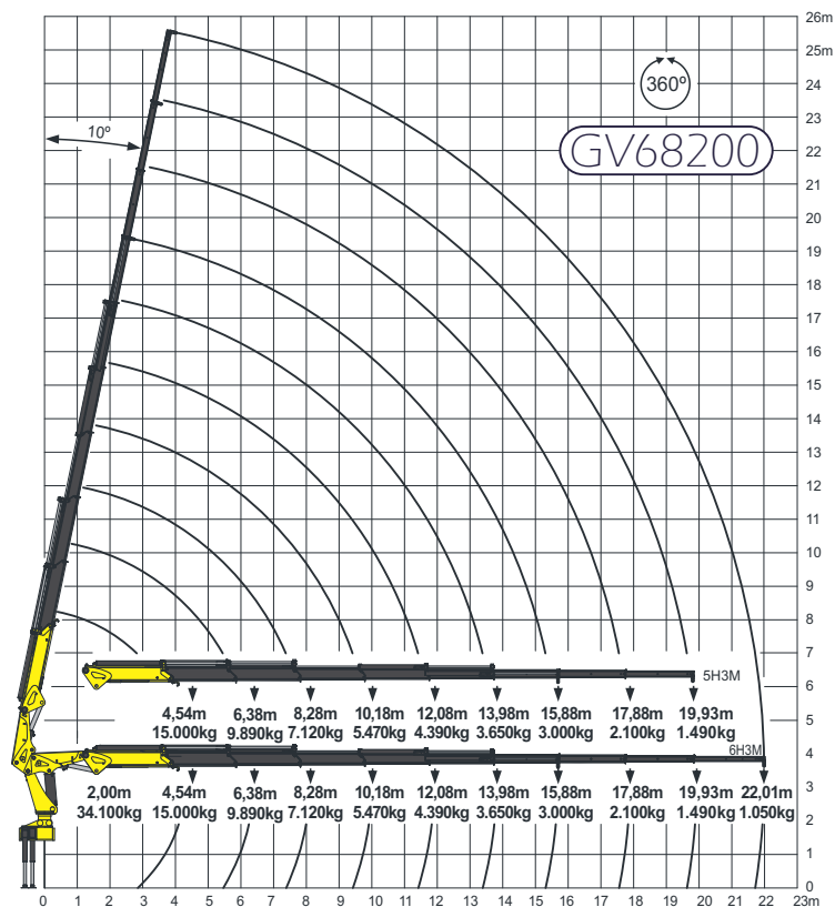
Gráfico de carga 6H3M e 5H3M
