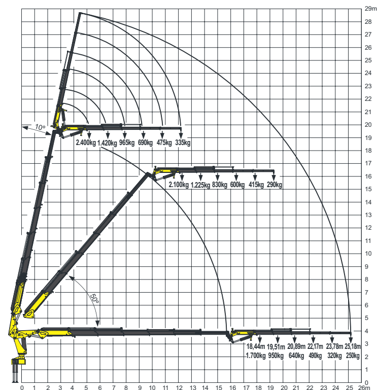
Gráfico de carga com Fly-Jib
