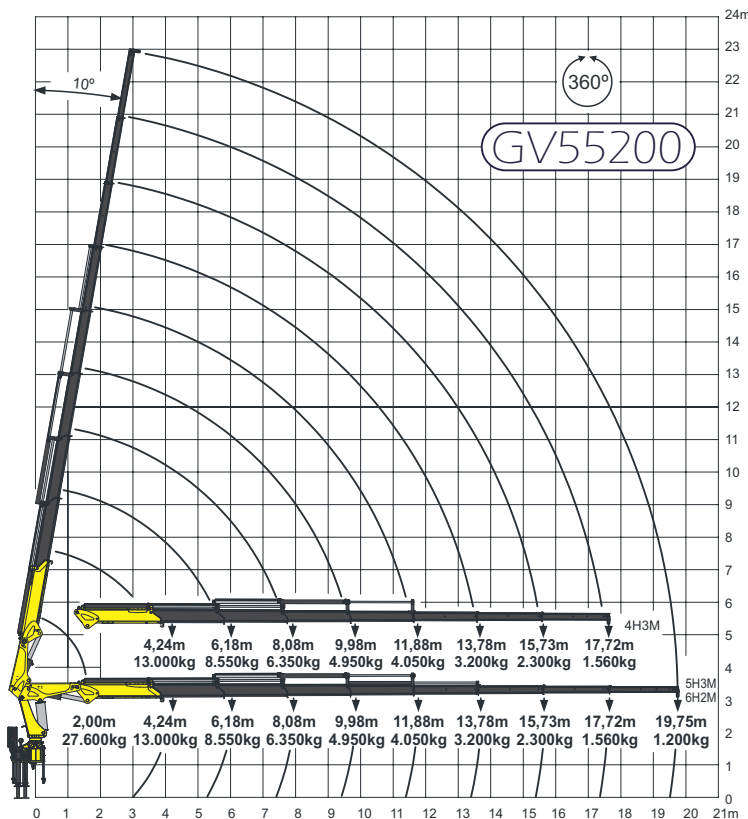
Gráfico de carga 6H2M, 5H3M e 4H3M
