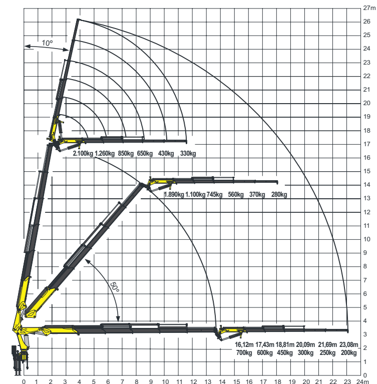
Gráfico de carga com Fly-Jib
